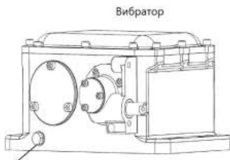
Масляная пробка вибратора
